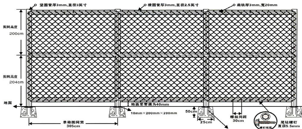
围网安装结构示意图
