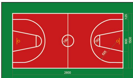
篮球场标线尺寸
