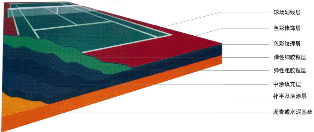
丙烯酸网球场施工
