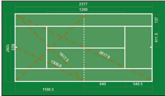
网球场标线尺寸
