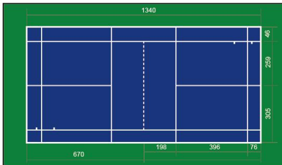
羽毛球场标线尺寸
